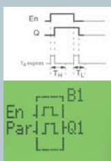
随机通/断定时器
