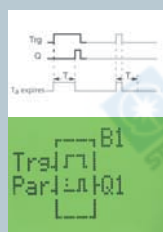
接通延时定时器
