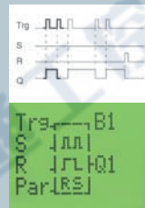
脉冲继电器
