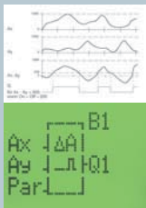
模拟量比较器
