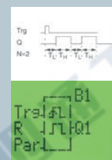
沿触发电宽继电器
