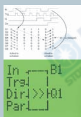
移位寄存器
