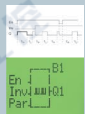
异步脉冲发生器
