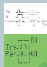
脉宽继电器 (脉冲输出)
