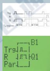
关断延时定时器
